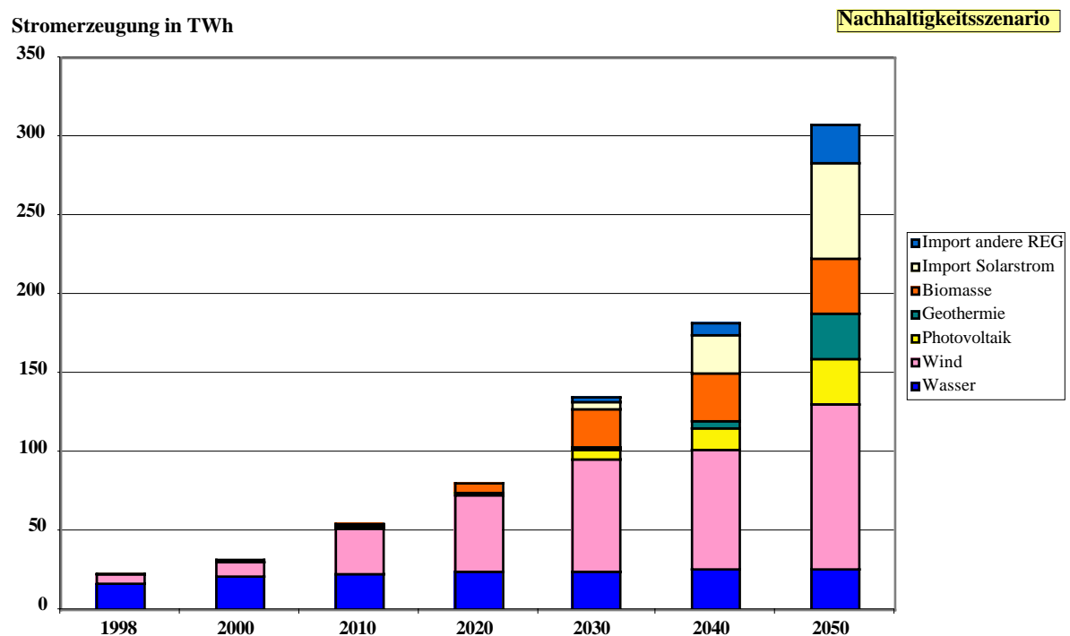
Abb. 2: Entwicklung der REG-Stromerzeugung im Nachhaltigkeitsszenario
